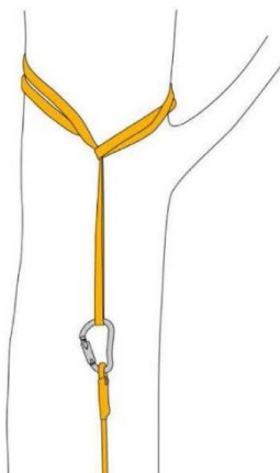
Fig. 5 - Ancoraggio della fune con dispositivo strozzo mediante anello di fettuccia
